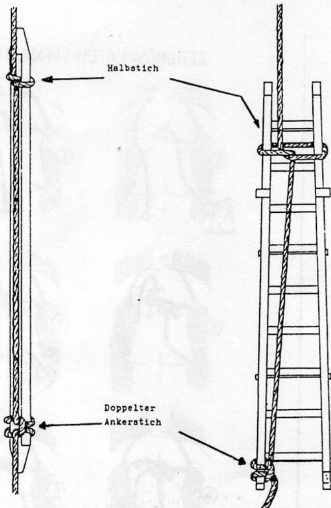
Abb. 21 Hochziehen der Klappleiter
